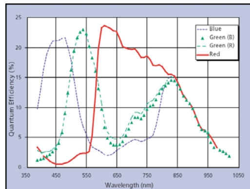
Abb. 2 spektrale Empfindlichkeit UK2001-C
