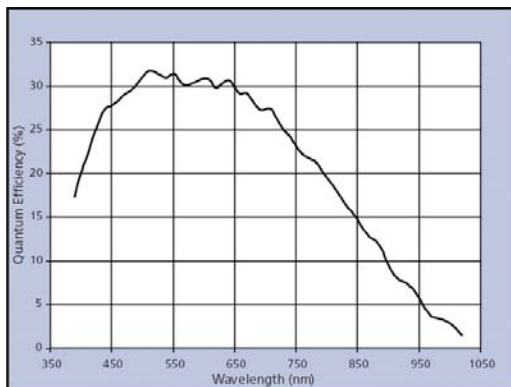
Abb. 1 spektrale Empfindlichkeit UK2001-M
